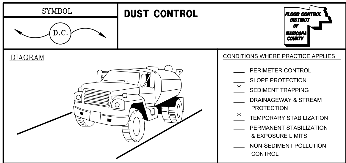
BMP DETAIL EC-7 N.T.S.
