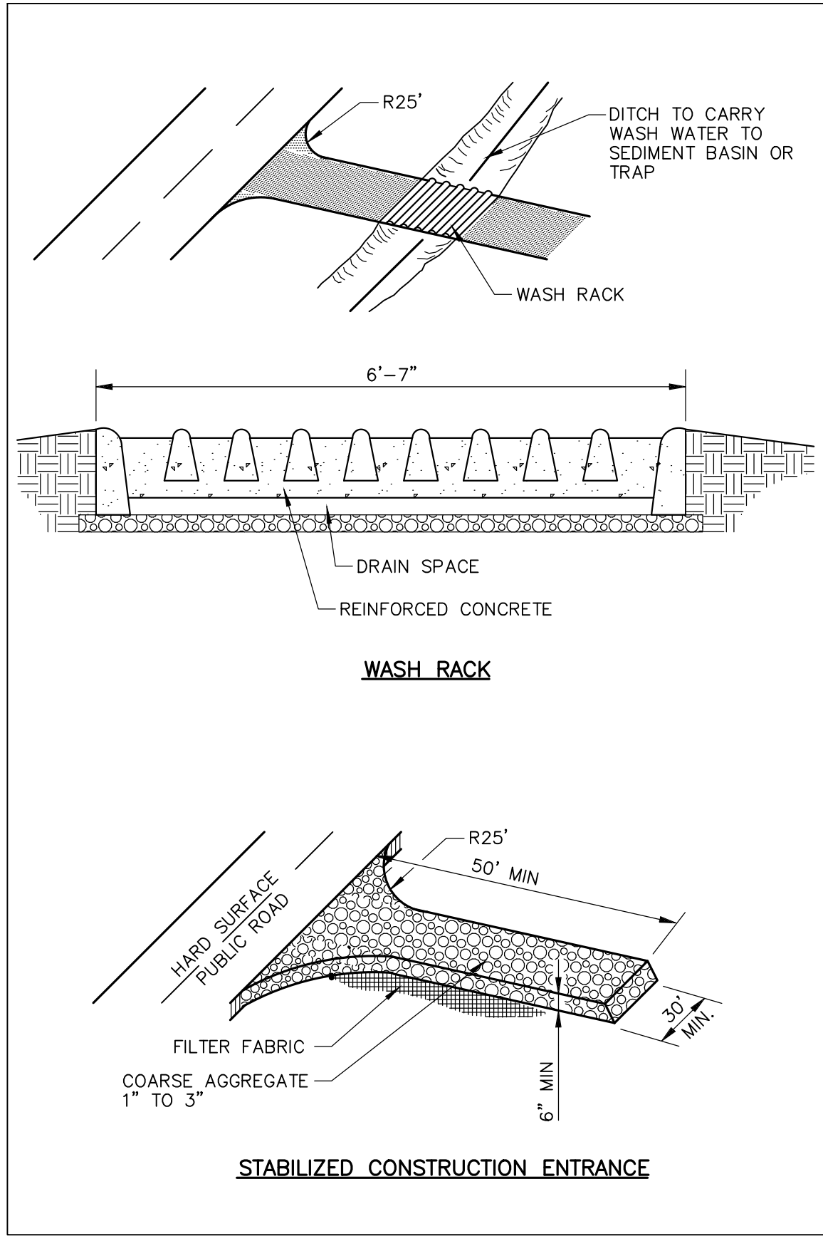
BMP DETAIL EC-5 N.T.S.
